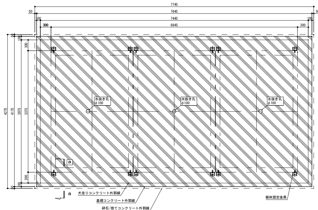
基礎伏図
