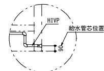
「給水管」接続口 詳細図
