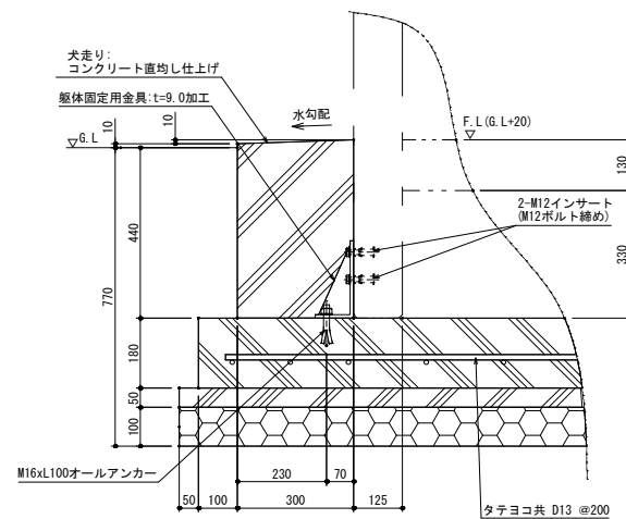
基礎部断面 詳細図 (a-a) Scale 1:10
