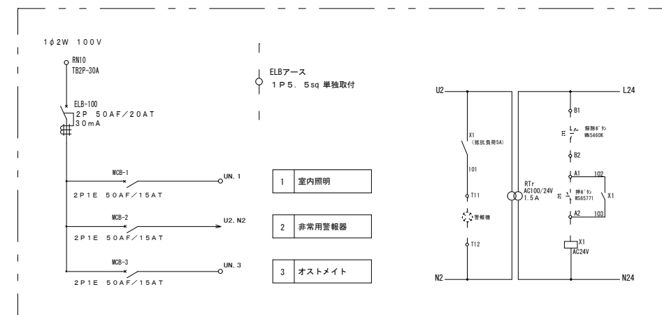
「分電盤」回路図 (参考)
