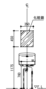
E 矢視図
