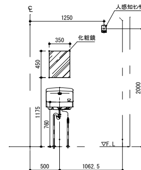
D 矢視図
