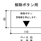
説明サインB 詳細図 Scale 1:3 アルミ複合板-110x60x3.0 インジエイト印刷 (UV74A貼リ)
