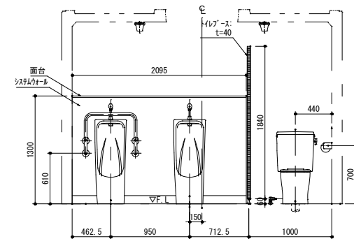
C-C 矢視図
