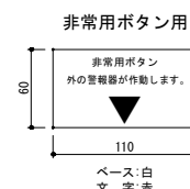
説明サインA 詳細図 Scale 1:3 アルミ複合板-110x60x3.0 インジエイト印刷 (UV74A貼リ)
