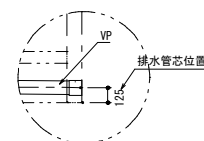
「排水管」接続口 詳細図
