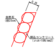
取付工 (練石積) S=1:20
