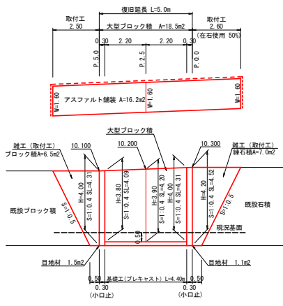
展開図 S=1:100
