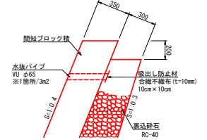
取付工 (ブロック積) S=1:20
