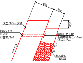
大型ブロック積 (S=1:0.4 控え50cm) S=1:20
