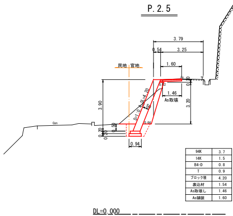
横断面 S=1:100
