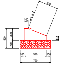
基礎工 (参考図) (S=1:0.4 控 50cm) S=1:20
