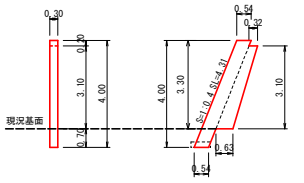
小口止工 S=1:100 P. 5.0
