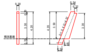
小口止工 S=1:100 P. 0.0
