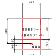
土工断面1
