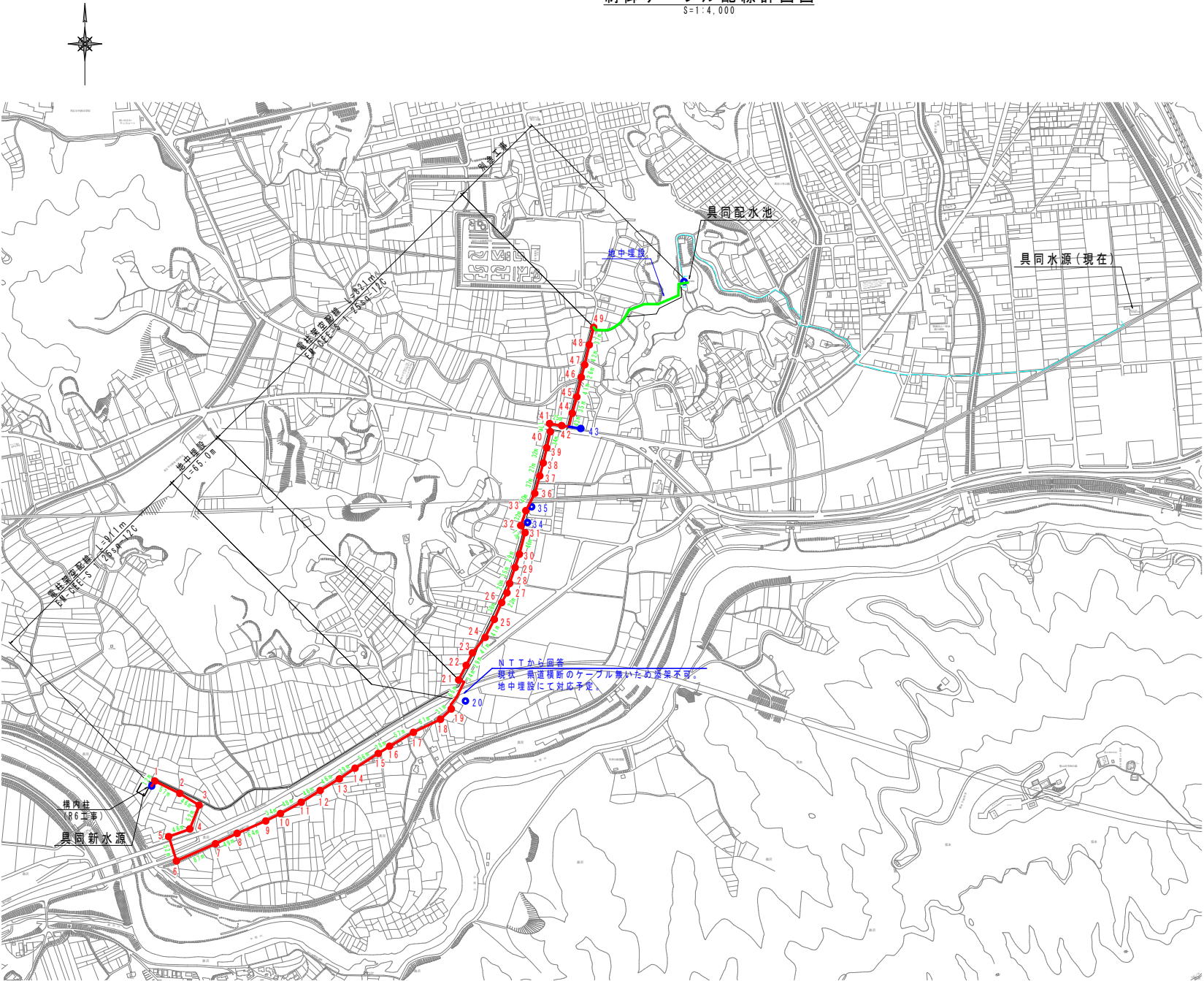
制御ケーブル配線計画図 S=1:4,000
