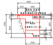
土工断面2
