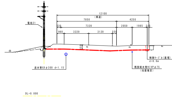
横断面 S=1:100 A-A
