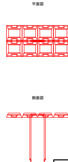
アンカーピン打設図
