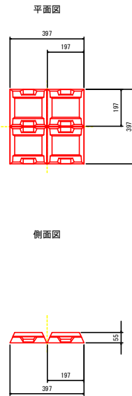
コンクリートブロック詳細図
