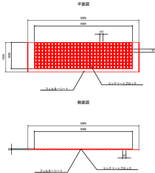
ブロックマット構造図
