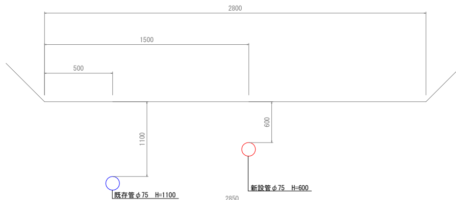
横断図B路線 1 (P. 5.0)
