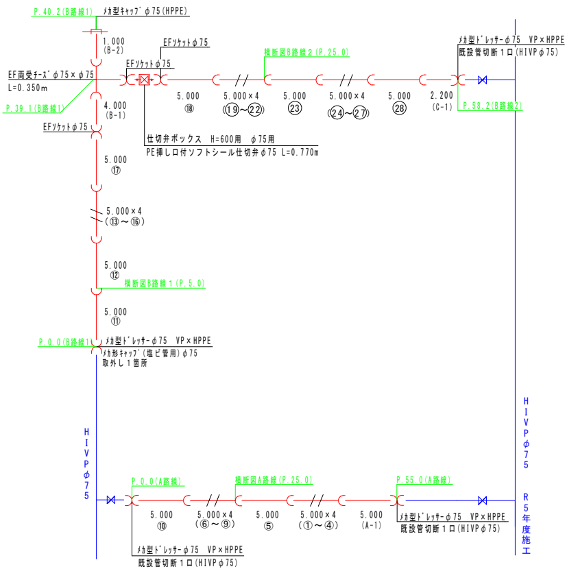
水道配水用φ75パイプ管切替調査 HPPEφ75:直管L=5,000m
