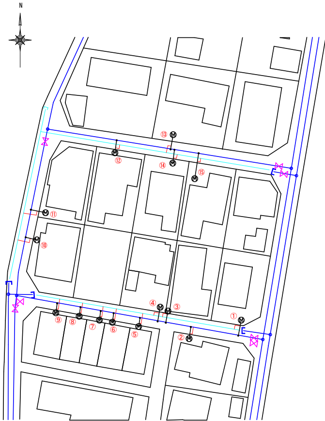
給水管接合替平面図 S=1:30
