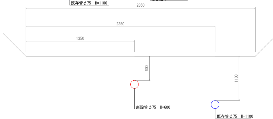
横断図B路線 2 (P. 25.0)
