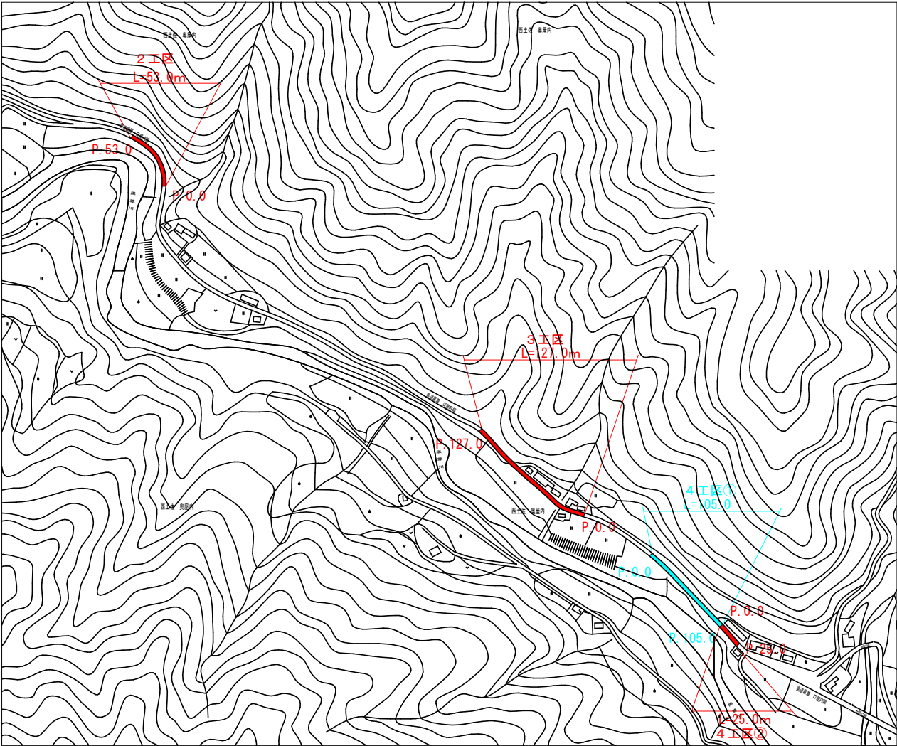
平面図 S=1:2000
