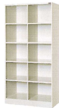
ZETF2-5N (2列5段 10人用) H1790×W900×D510 ※ZAM鋼板仕様
