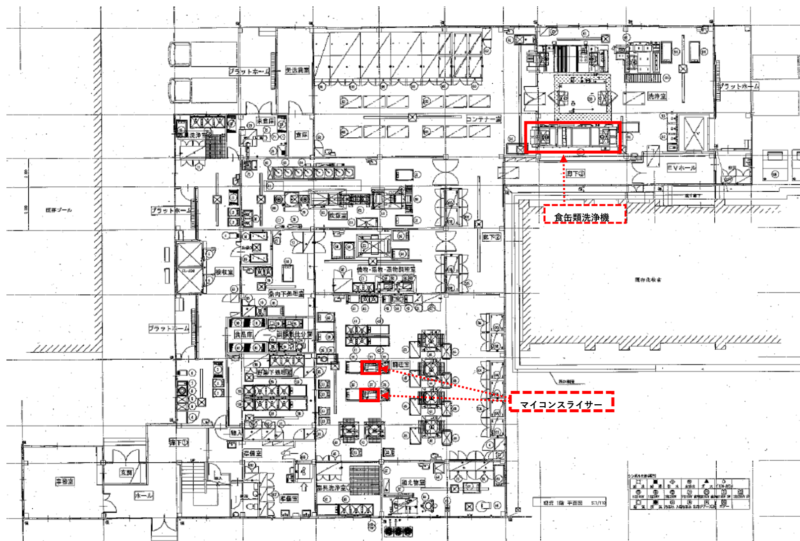
スクールミールなかむらみなみ厨房機器図面
